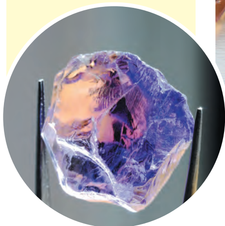
Аметрин, минерал
